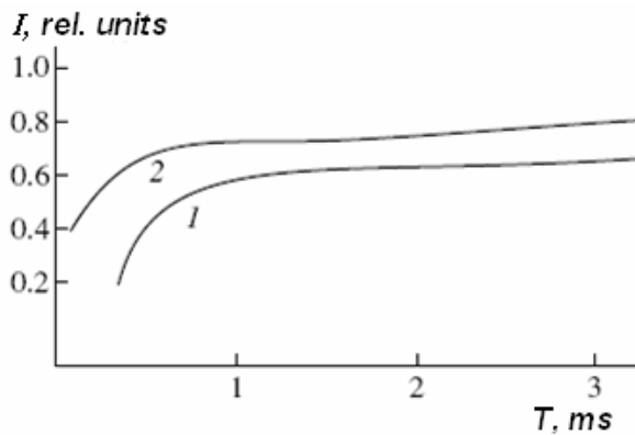
ნახ. 14. \text{Co}_2\text{MnSi} -ში ^{59}\text{Co} –ბირთვებზე ორიმუდსიანი (2) და ერთიმუდსიანი (1) ექოს ინტენსივობების დამოკიდებულება განმეორების T პერიოდზე.
